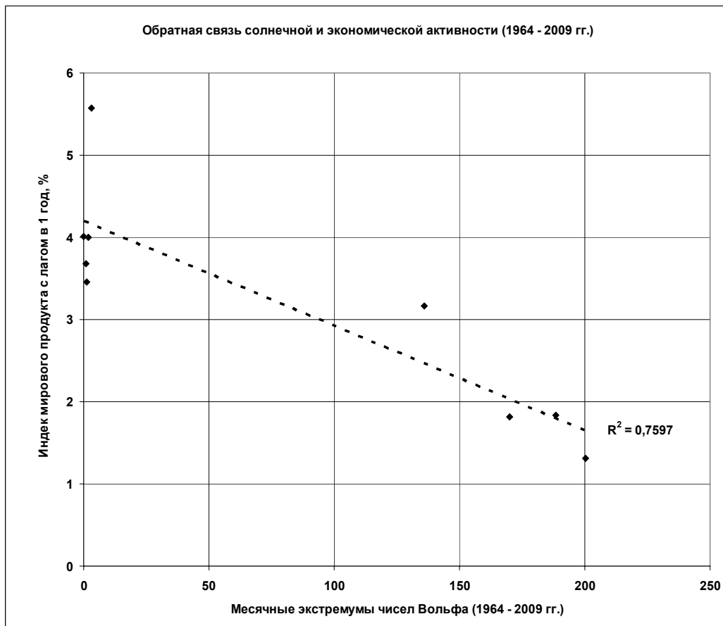
Рис. 4. Сильная обратная связь месячных экстремумов чисел Вольфа и годовых темпов роста мирового продукта с лагом в 1 год
