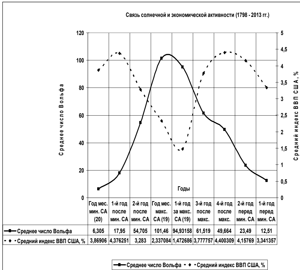
Рис. 2. Циклы Китчина и Жюгляра ВВП США как функция солнечной активности (1798–2013 гг.)
