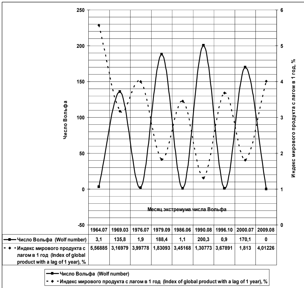
Рис. 3. Сильная обратная связь циклов мирового продукта и циклов солнечной активности
